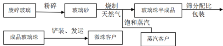
图 1-1 生产工艺流程图
